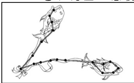
「うお座」ステラナビゲータより
